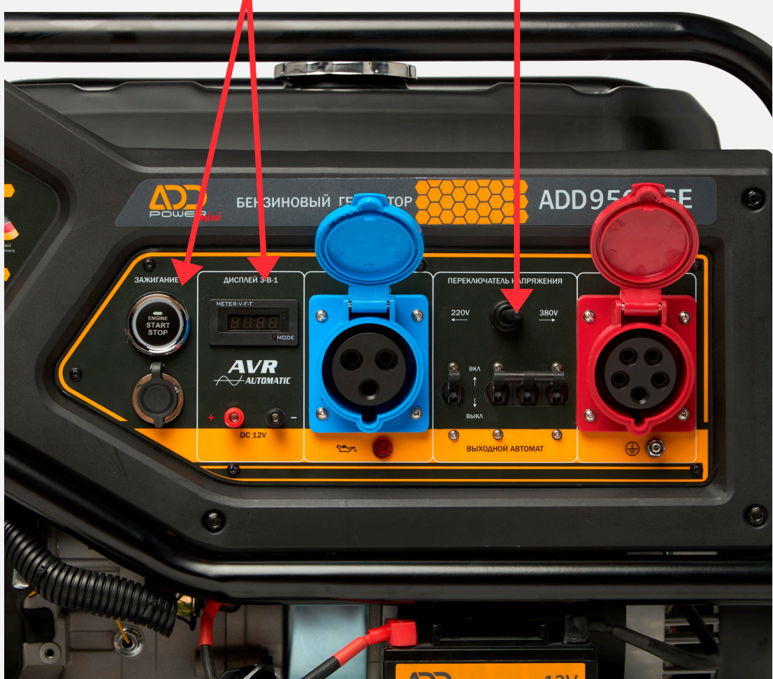
Панель управления
